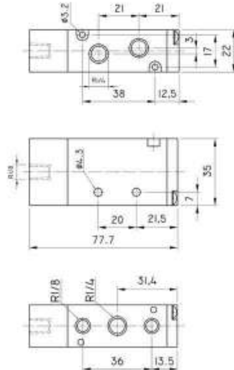
PY - 52 1/4 eco
