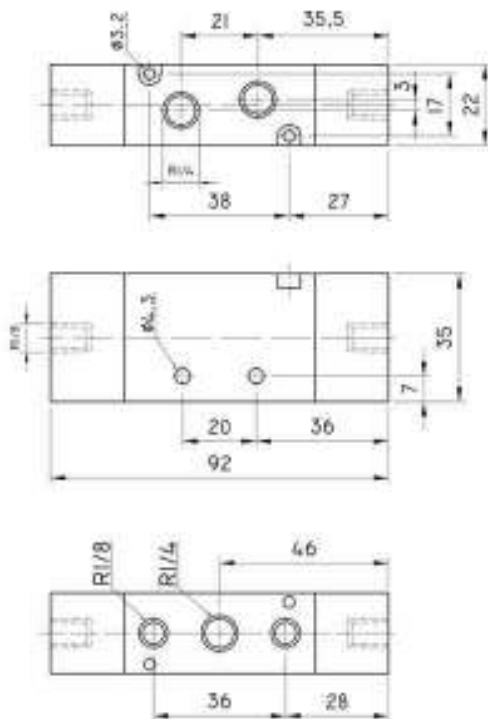
PP - 52 1/4 eco
