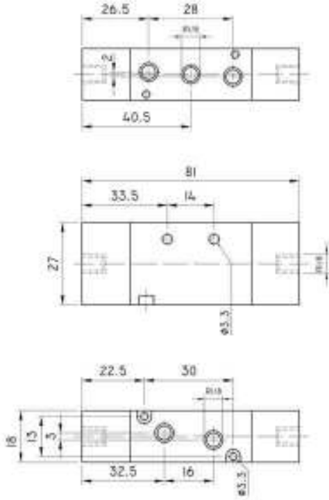
PP - 52 - 1/8 eco
