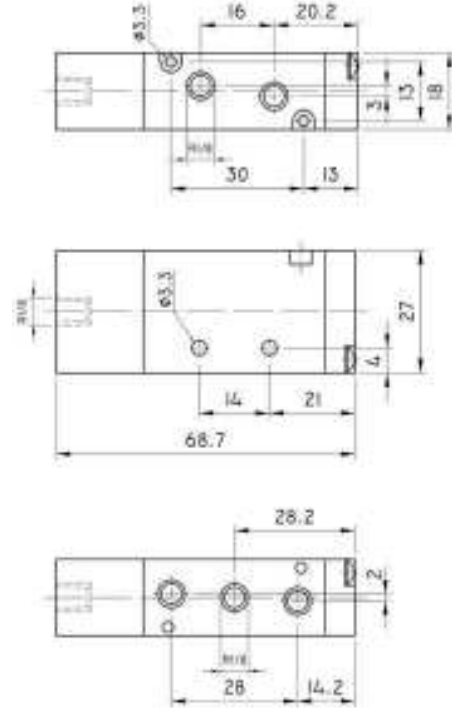
PY - 52 - 1/8 eco
