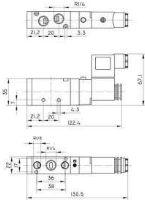
ESY - 52 - 1/4 eco
