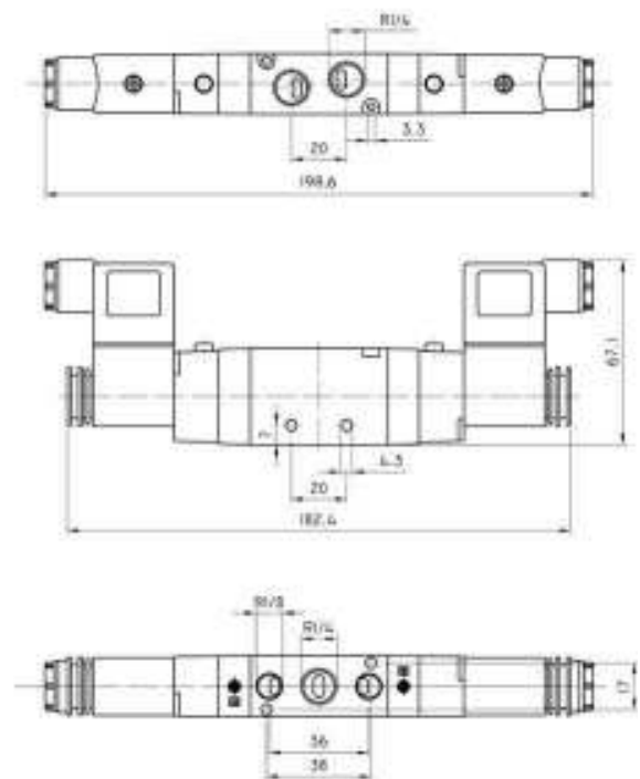
EES - 52 - 1/4 eco
