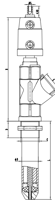
回吸灌装阀结构简图
