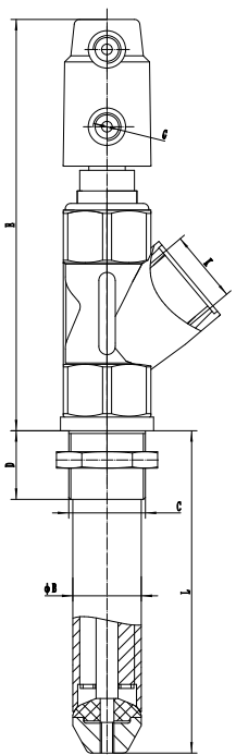
外封灌装阀结构简图
