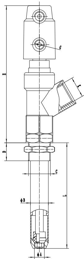
内封灌装阀结构简图
